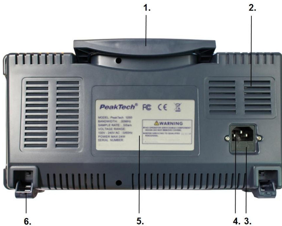
Abb. 3 Rückseite des Oszilloskops
