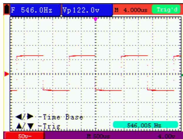
Abbildung 39: Punktanzeige
