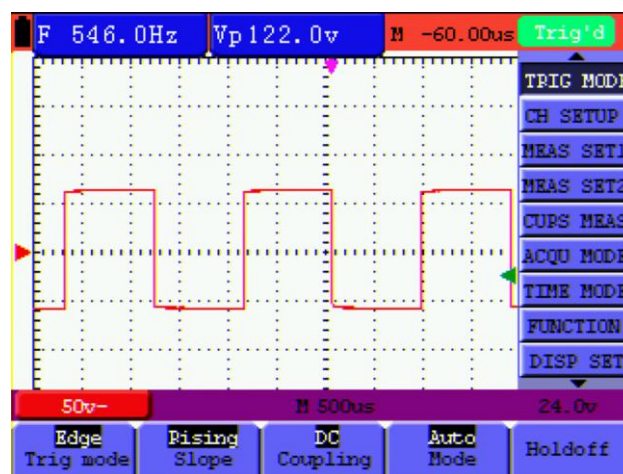
Abbildung 34: Flanken-Trigger
