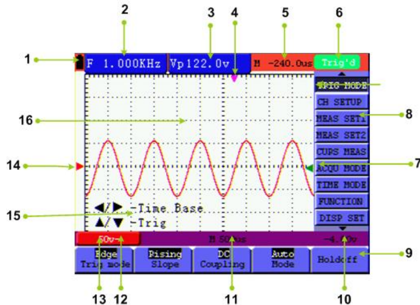
Abbildung 4: Oszilloskop Betriebsanzeige
