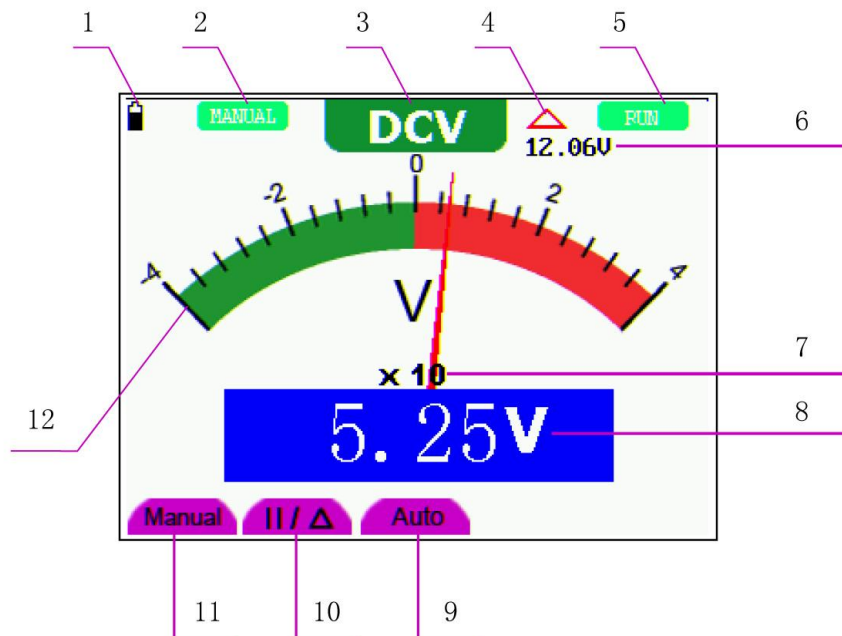
Abbildung 16: Betriebsanzeige DMM
