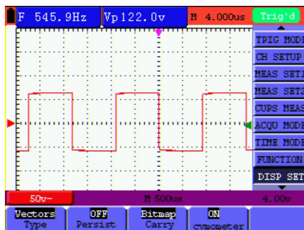
Abbildung 40: Vektoranzeige
